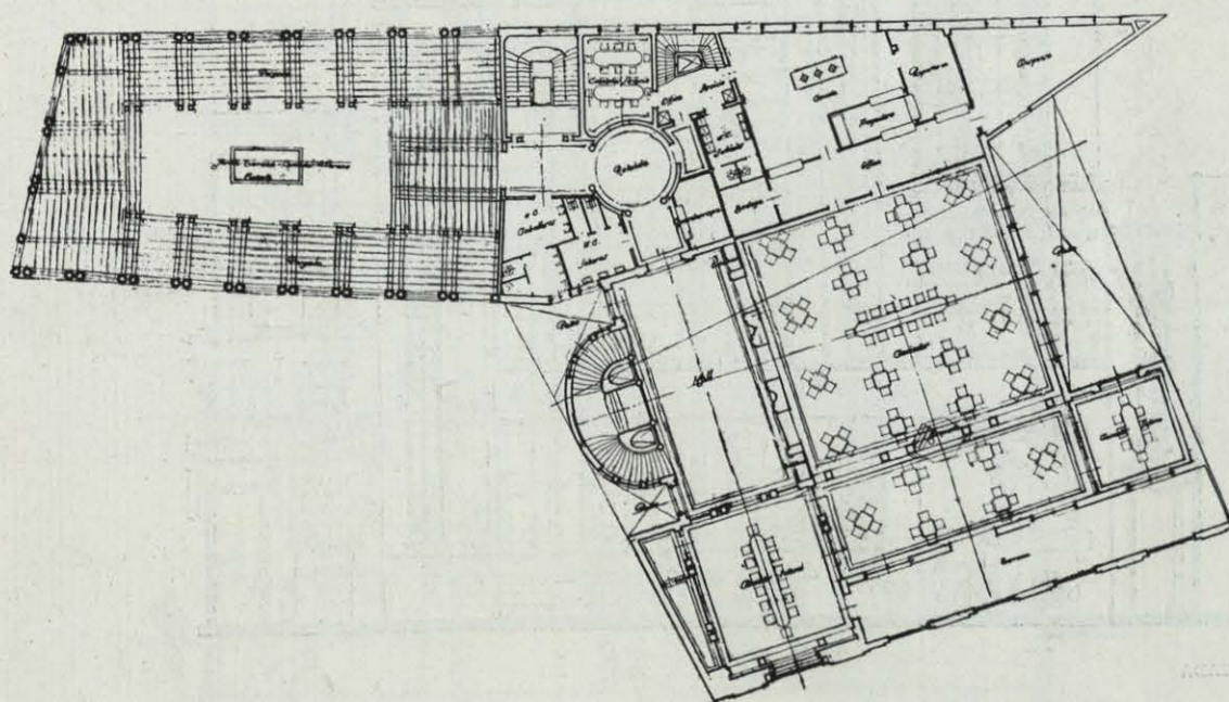
PLANTA QUINTA.
