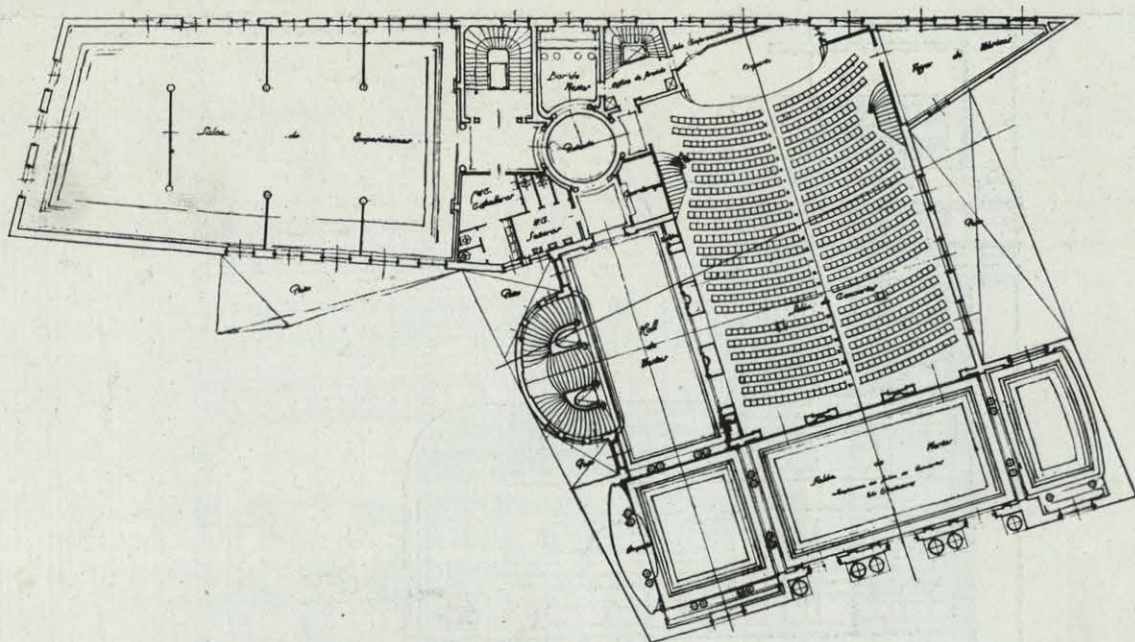
PLANTA SEGUNDA.
